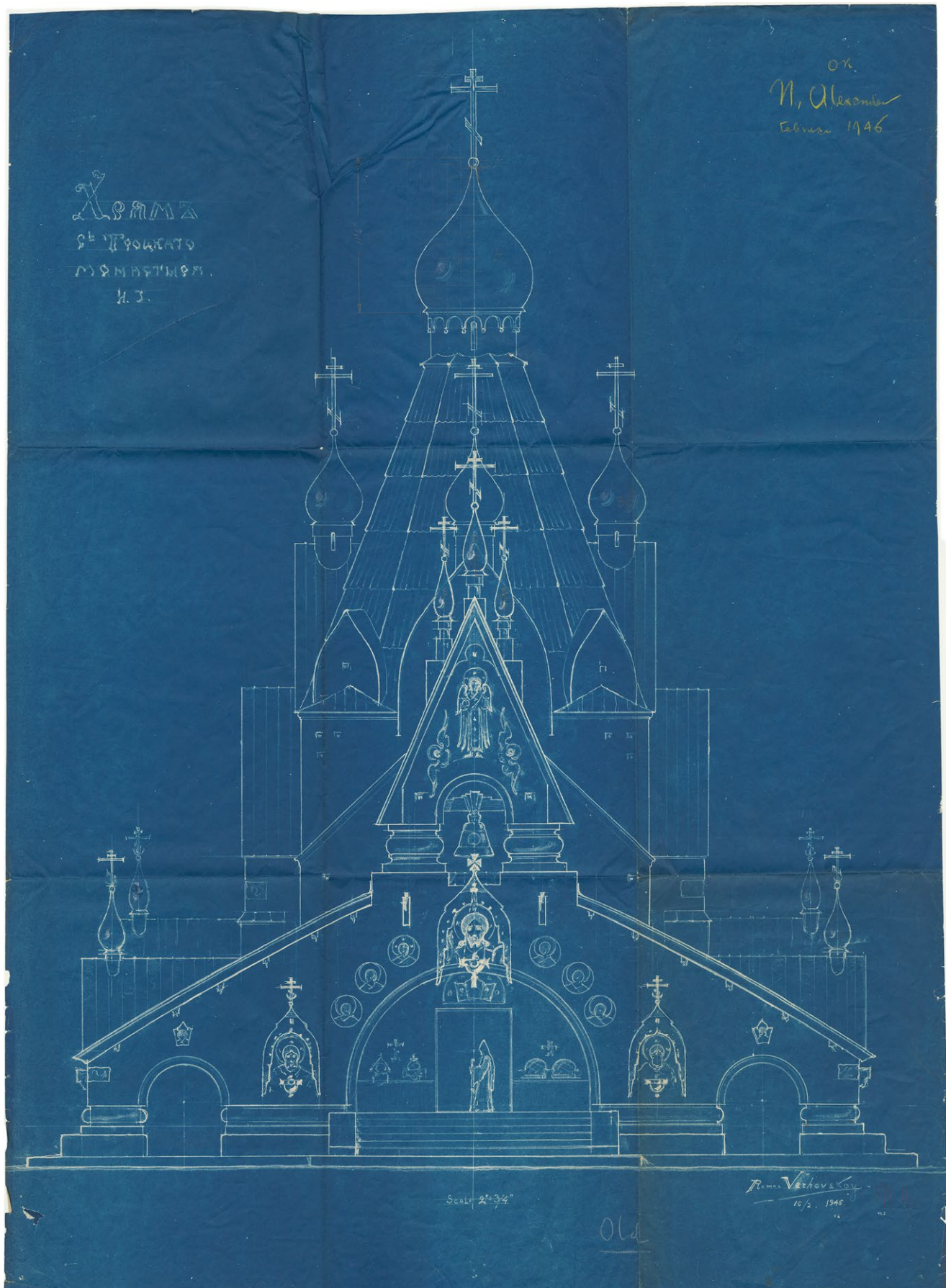
Окончательный проект главного храма Свято-Троицкого монастыря. Надпись на оборотъ: «Этотъ проектъ, выполненный правильно къ построению будетъ оцѣненъ по достоинству если не заказчикомъ, то послѣдующими поколѣніями. 1946».
