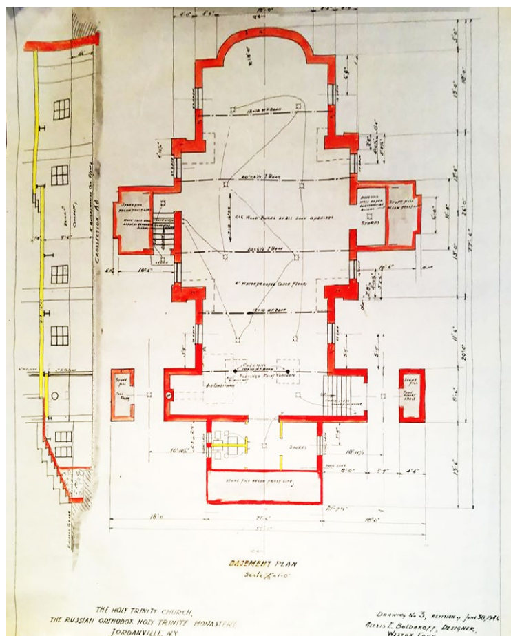
Чертежи А. Е. Болдакова
